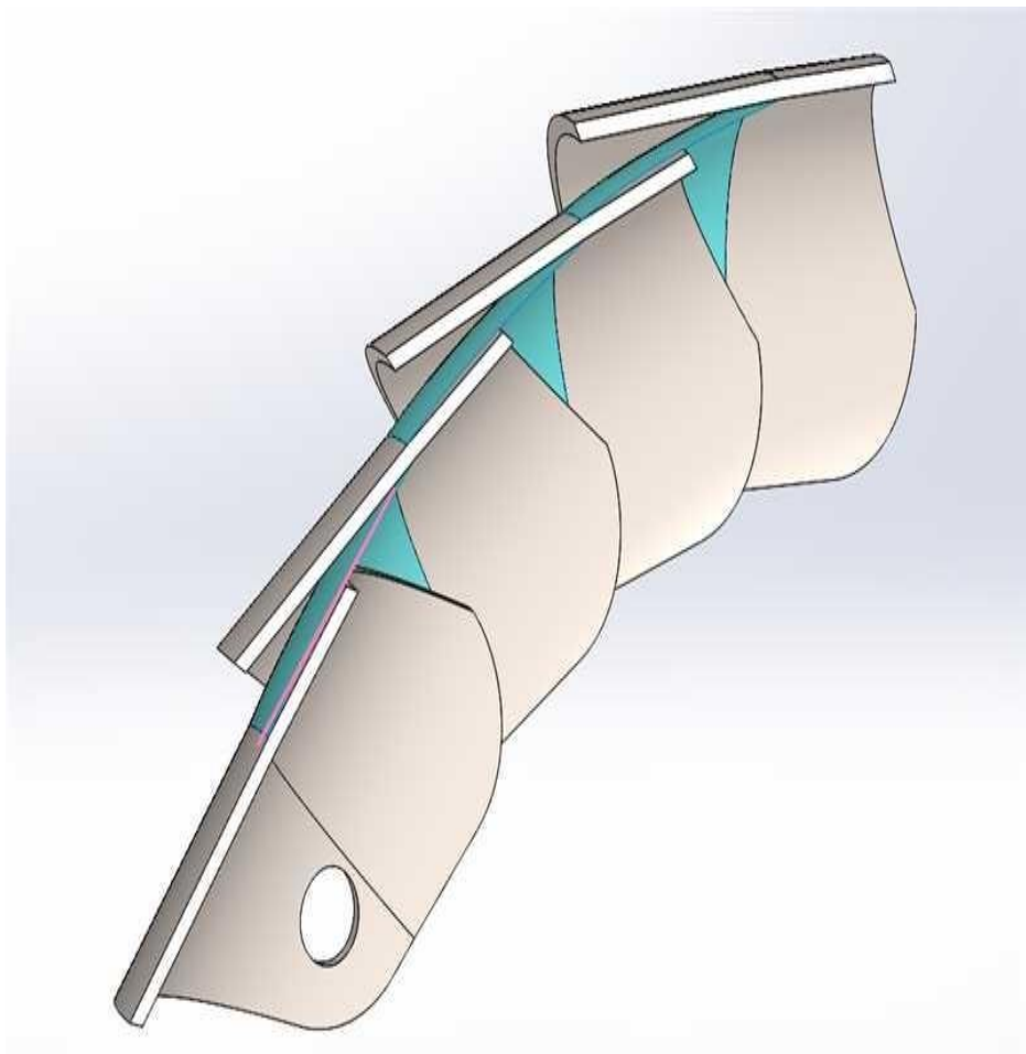
虾壳式多段关节完整 CAD 模型
