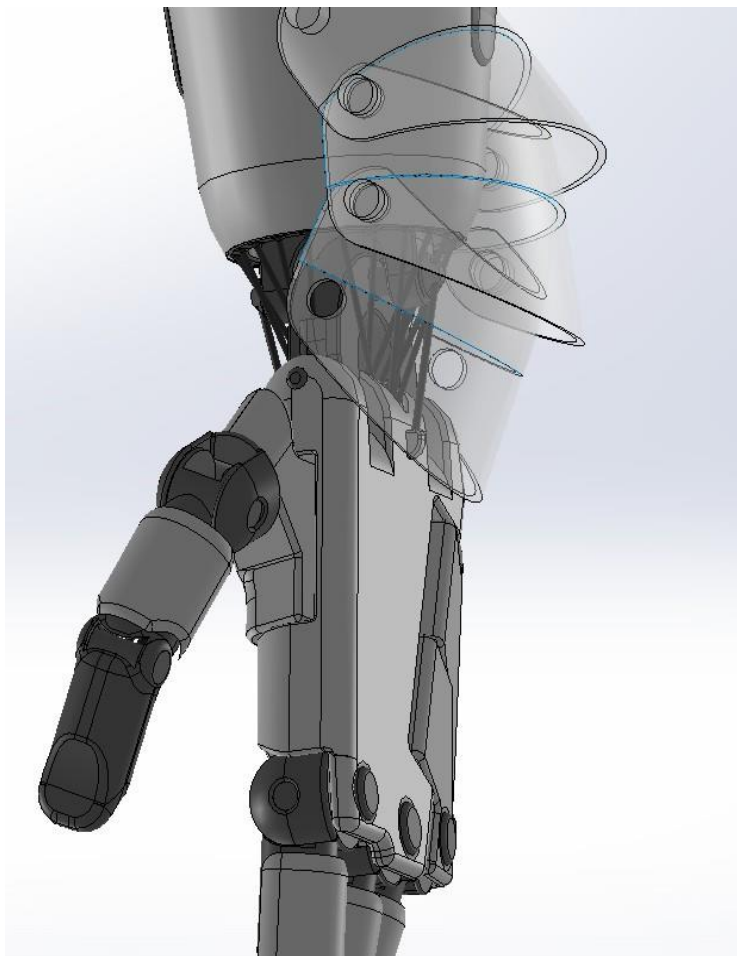
虾壳式多段关节完整 CAD 模型 前视图
